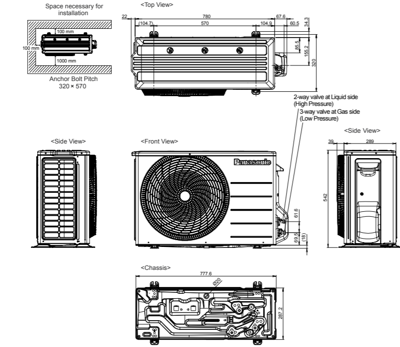
Dimensions (2.5kW – 2.6kW) CU-Z25UBRA
